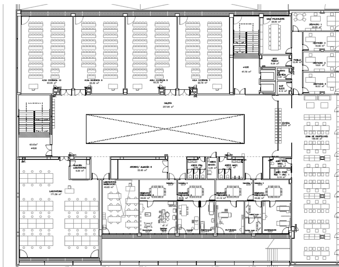
Ilustración 5: Plano planta 2 Edificio CREAR
