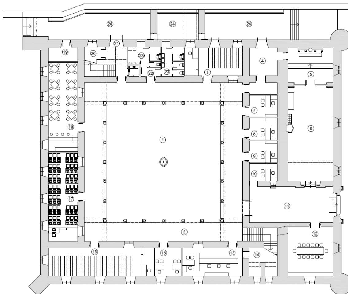
Ilustración 1: Plano planta baja Edificio Principal
