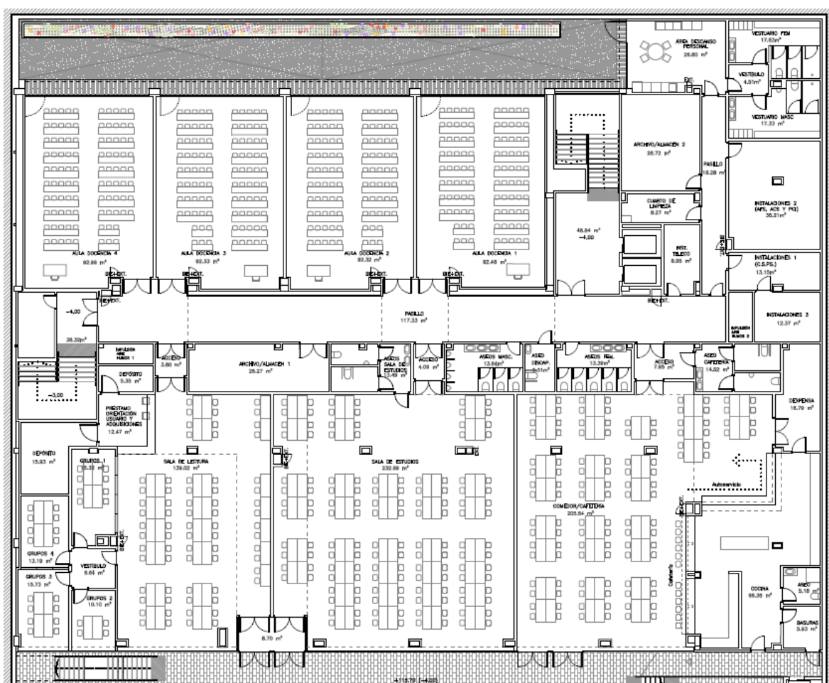
Ilustración 3: Plano planta 0 Edificio CREAR
