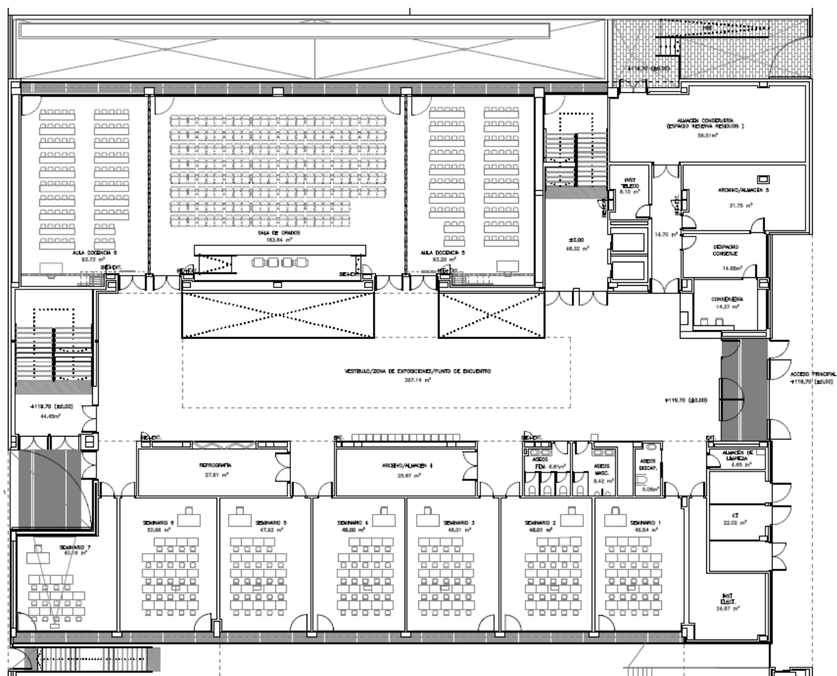
Ilustración 4: Plano planta 1 Edificio CREAR
